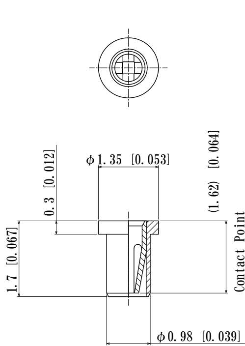
NZP-F135L17-GG
